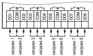
Рисунок 6 – Подключение нагрузки к ВЭ типа «Р»
