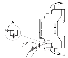
Рисунок 3 – Отсоединение съемных частей клемм
