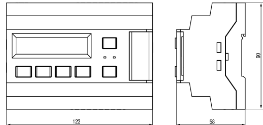
Рисунок 2 – Габаритный чертеж прибора
