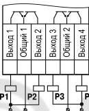
Рисунок 10 – Схема подключения нагрузок типа «КТ»
