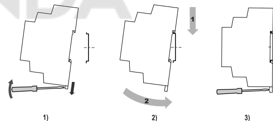
Рисунок 1 – Монтаж прибора
