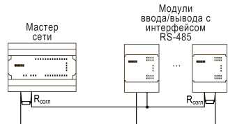
Рисунок 12 – Типовая схема подключения в режиме Master
