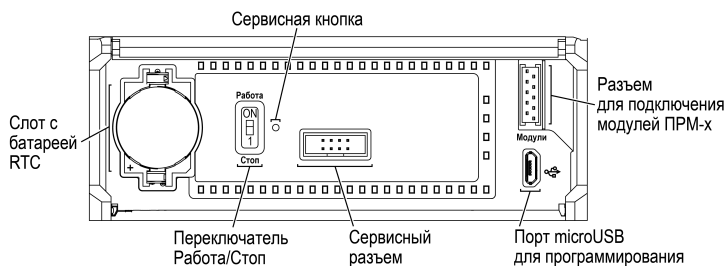
Рисунок 16 – Лицевая панель под крышкой
