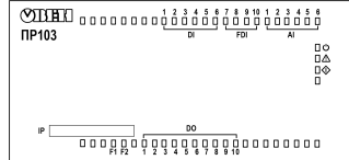
Рисунок 16 – Пример лицевой панели прибора
