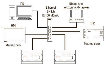
Рисунок 14 – Подключение по схеме «Звезда»
