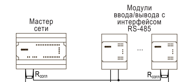
Рисунок 13 – Типовая схема подключения в режиме Master
