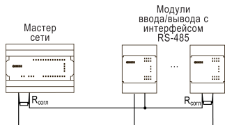
Рисунок 11 – Типовая схема подключения в режиме Master
