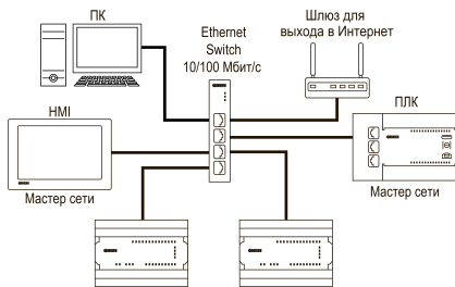
Рисунок 12 – Подключение по схеме «Звезда»
