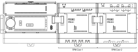
Рисунок 7 – Расположение модулей расширения на шине
