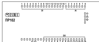
Рисунок 8 – Лицевая панель прибора
