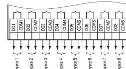
Рисунок 4 – Схема подключения нагрузок к ВЭ типа «Р»
