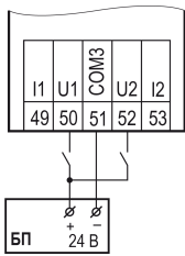
Рисунок 6 – Схема подключения к универсальным входам, работающим в дискретном режиме датчиков типа «сухой» контакт
