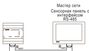
Рисунок 11 – Типовая схема подключения для PR100 в режиме Slave
