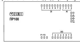
Рисунок 13 – Лицевая панель прибора
