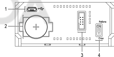
Рисунок 14 – Лицевая панель под крышкой
