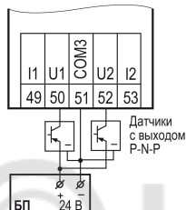
Рисунок 7 – Схема подключения к универсальным входам, работающим в дискретном режиме трехпроводных дискретных датчиков, имеющих выходной транзистор р-п-р-типа с открытым коллектором
