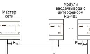
Рисунок 7 – Типовая схема подключения для PR100 в режиме Master
