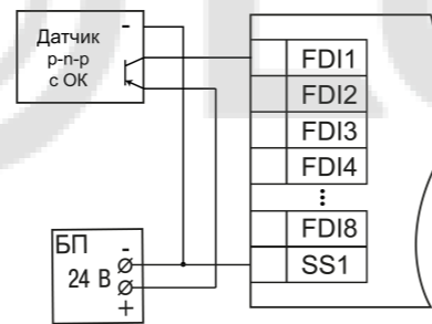
Рисунок 12 – Подключение транзисторов типа р-р-р
