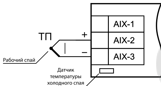
Рисунок 3 – Схема подключения термоэлектрического преобразователя
