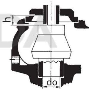
Высота подъема седла h
