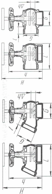
Рисунок 1—Внешний вид клапанов угловых моделей КПЛ, КПЧ, КПС и КПЛМ, КПЧМ, КПСМ Исполнение 1: КПЛ, КПЧ, КПС, КПСМ Исполнение 2: КПЛМ, КПЧМ, КПСМ
