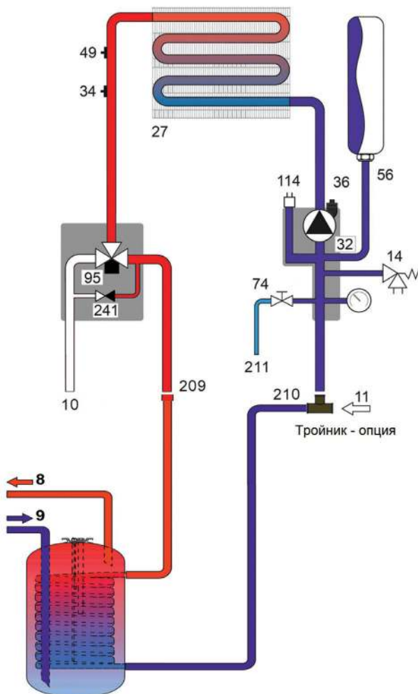
Рис. 19. Схема подключения внешнего бойлера
