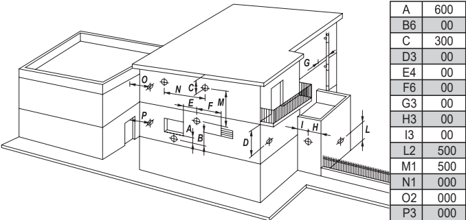
Рис. 11. Варианты расположения оголовка дымохода
