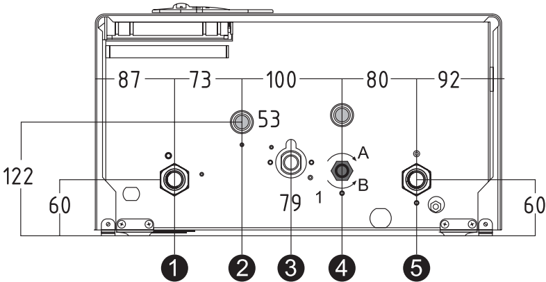
Рис. 21. Расположение штуцеров присоединения Vitabel HF13-40 кВт 1. Поддача в систему отопления. 2. Поддача на нагрев бойлера. 3. Вход газа. 4. Подпитка системы отопления. 5. Возврат из системы отопления/бойлера.
