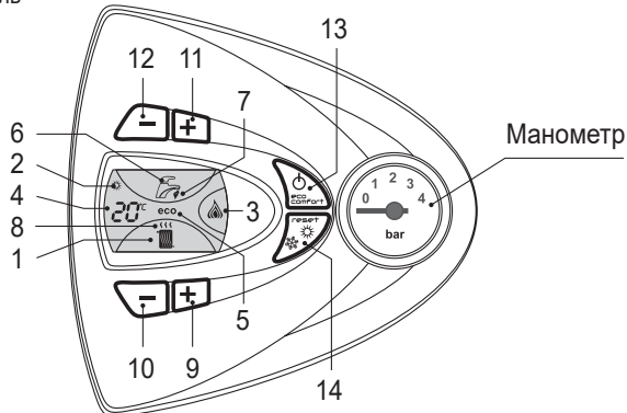
Рис. 1. Панель управления
