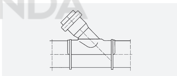
РИС. 15. ПРИКЛЕИВАЕМАЯ НАКЛАДКА С РАСТРУБОМ
