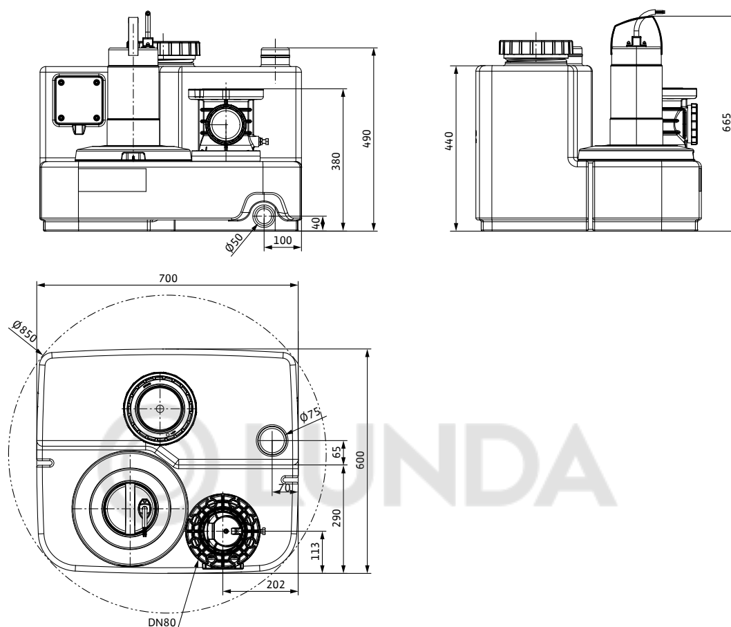
Габаритный чертеж DrainLift SANI-M.12 .../M.16 .../M.21 ...
