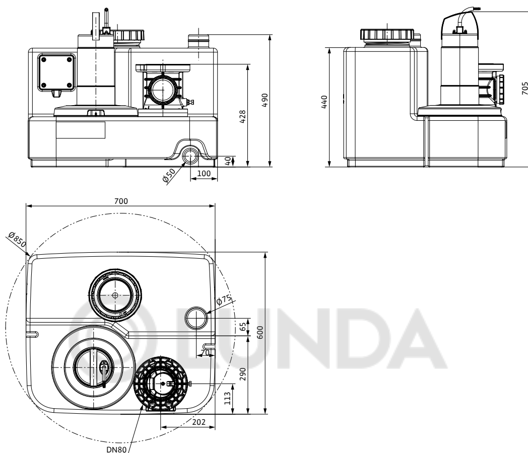
Габаритный чертеж DrainLift SANI-M.11 .../М.17 .../М.19 .../М.23 ...
