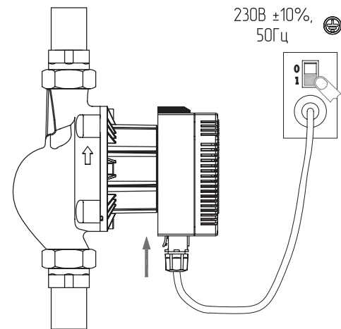
Рис. 36 Электроподключение насоса
