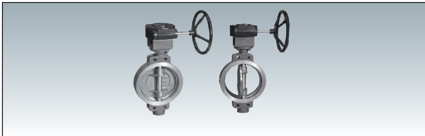
Поворотный затвор Ду 200 типа 161.155 с межфланцевым соединением
