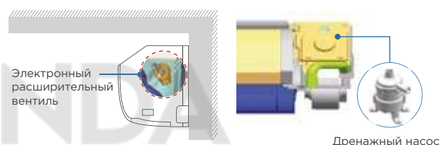
Дренажный насос
