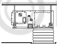
Для гибкого подсоединения к воздухозаборной панели (не поставляется Daikin)
