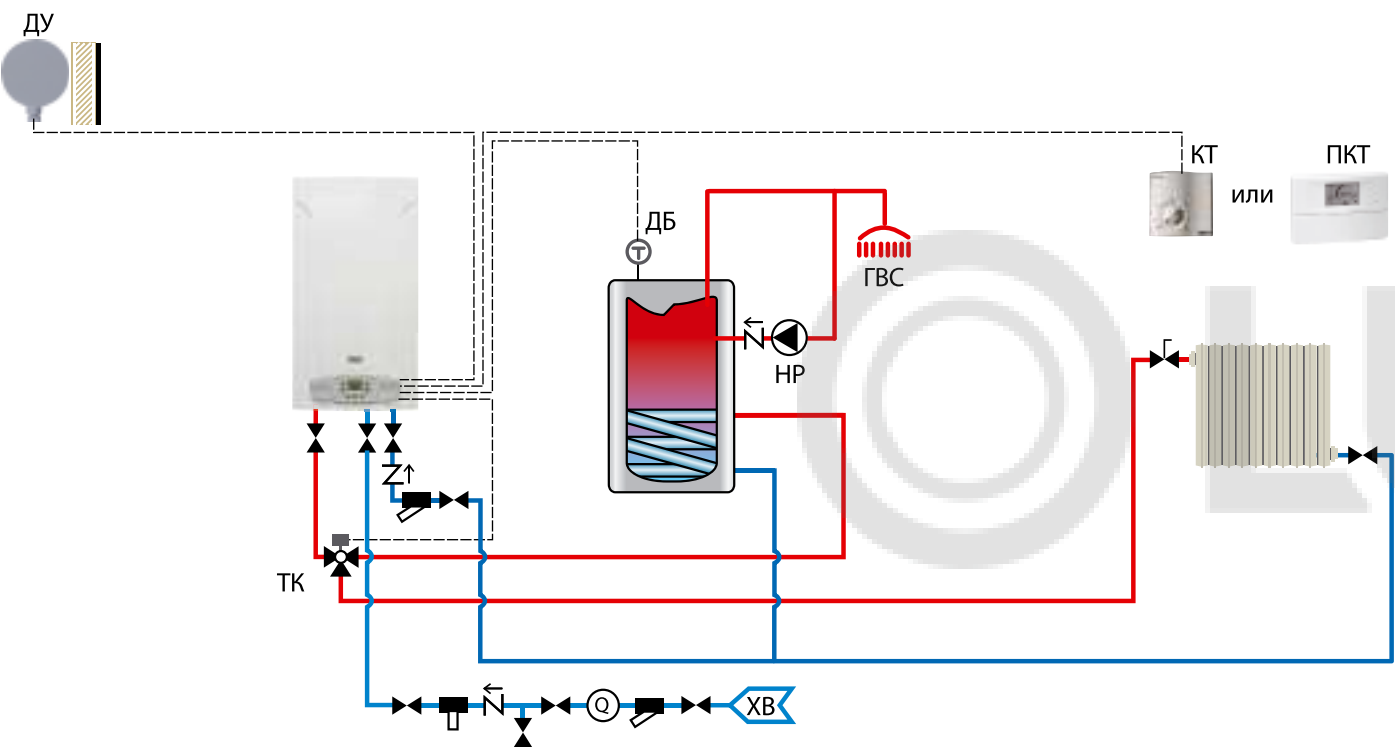
СХЕМА ОДИНОЧНОЙ УСТАНОВКИ КОТЛА ECO FOUR С БОЙЛЕРОМ ГВС И ОДНИМ ПОГОДОЗАВИСИМЫМ КОНТУРОМ ОТОПЛЕНИЯ
