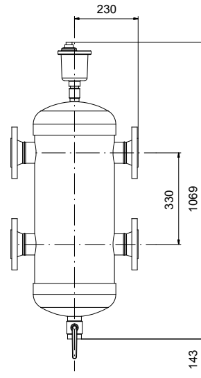
Гидравлический разделитель DN65
