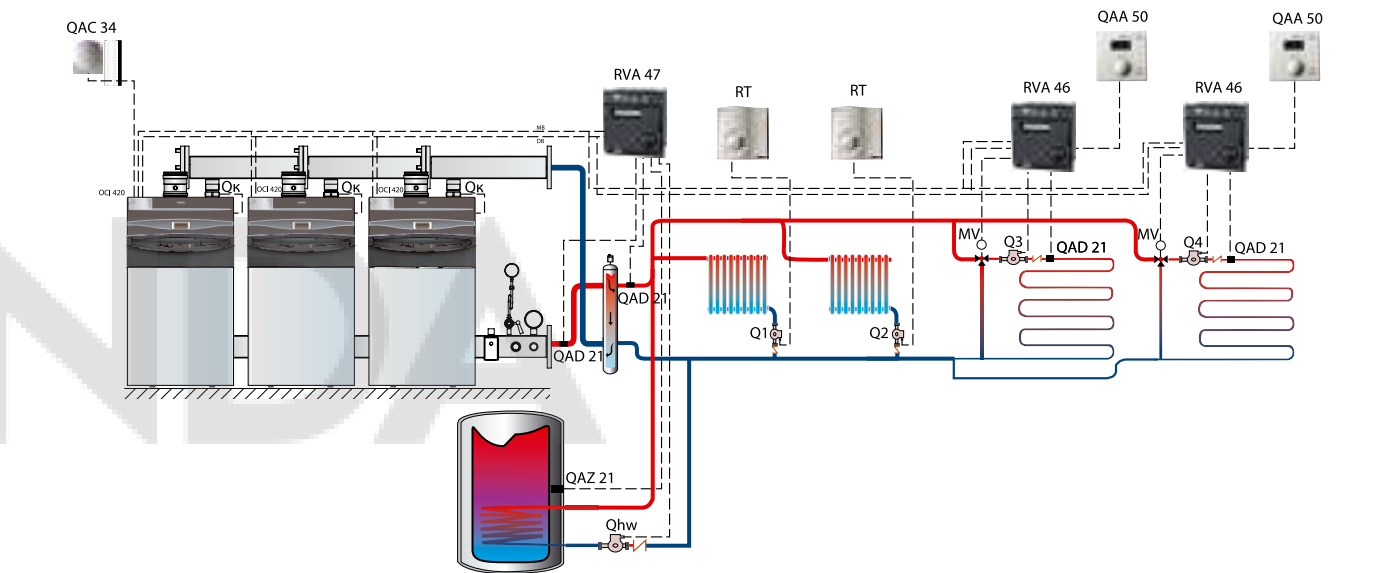
Схема каскадной установки котлов POWER HT с бойлером ГВС, двумя прямыми и двумя смесительными контурами отопления
