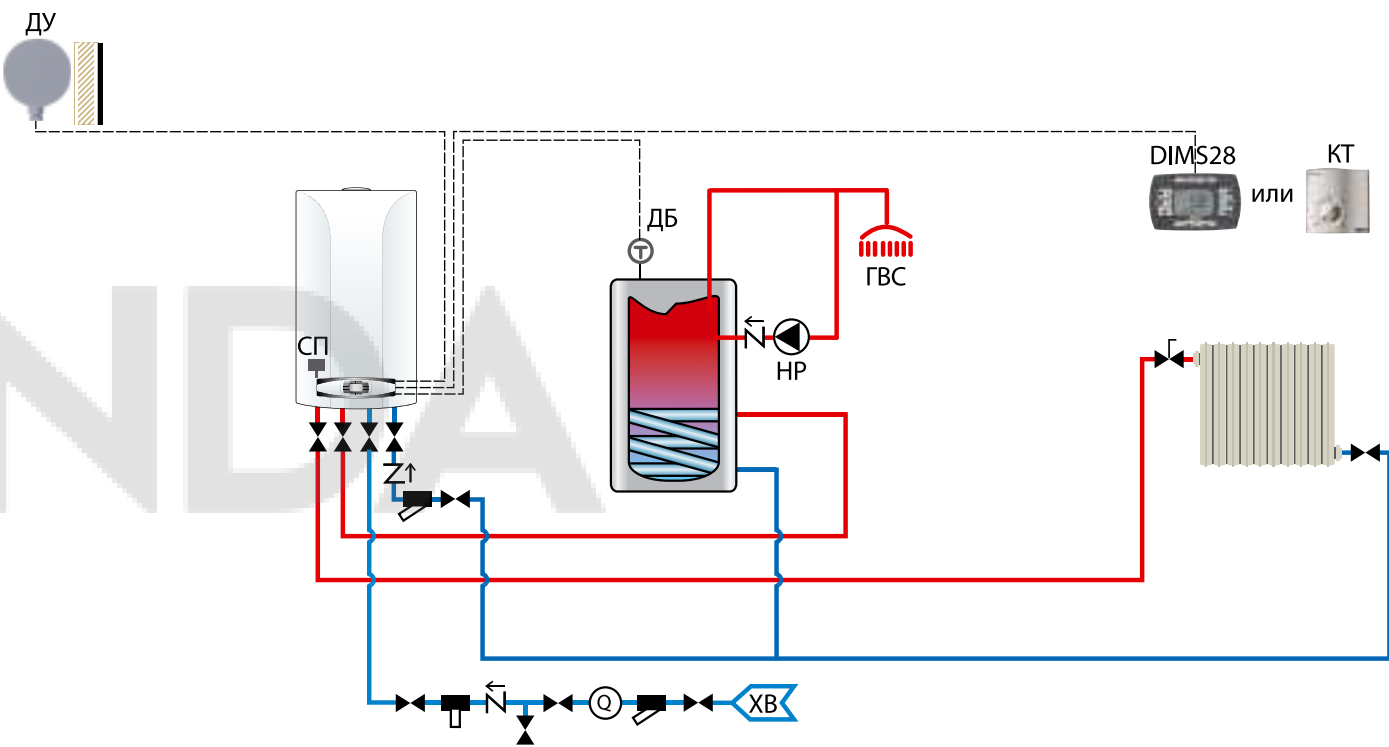
СХЕМА ОДИНОЧНОЙ УСТАНОВКИ КОТЛА LUNA-3 С БОЙЛЕРОМ ГВС И ОДНИМ ПОГОДОЗАВИСИМЫМ КОНТУРОМ ОТОПЛЕНИЯ
