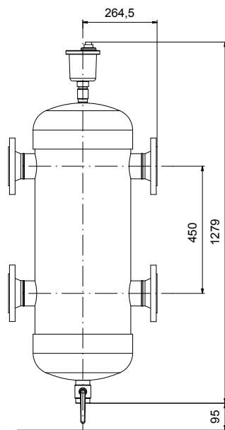
Гидравлический разделитель DN100
