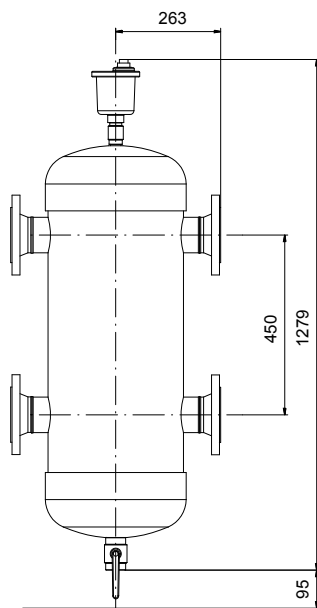
Гидравлический разделитель DN80
