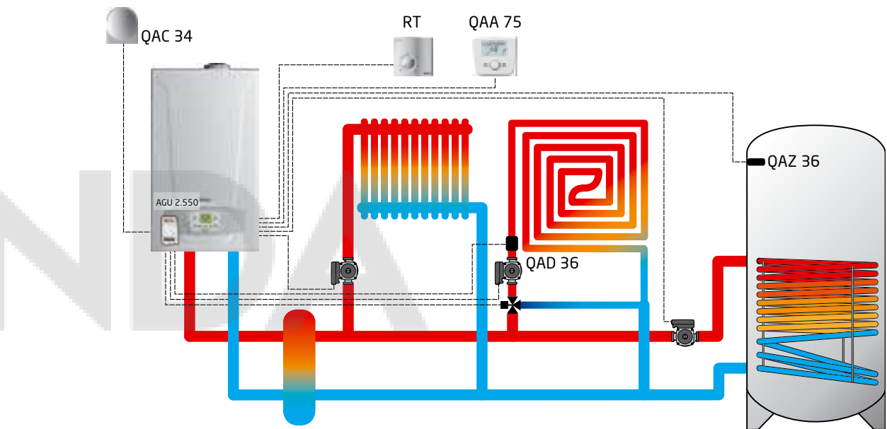
Схема одиночной установки котла LUNA Duo-tec MP с одним прямым контуром, одним смесительным контуром и бойлером ГВС
