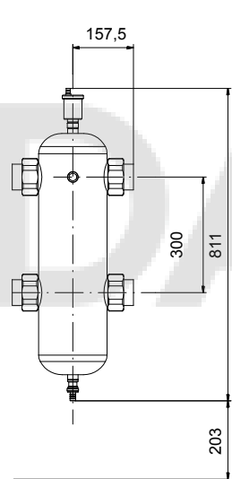
Гидравлический разделитель 2"
