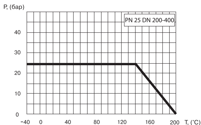
График «Температура-Давление»
