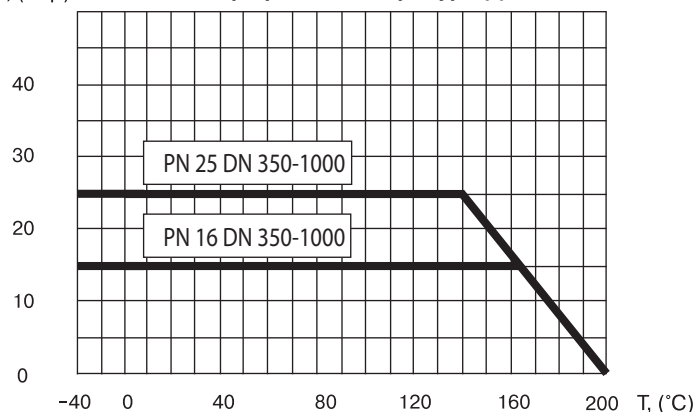
График «Температура-Давление»
