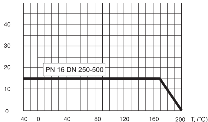
График «Температура-Давление»
