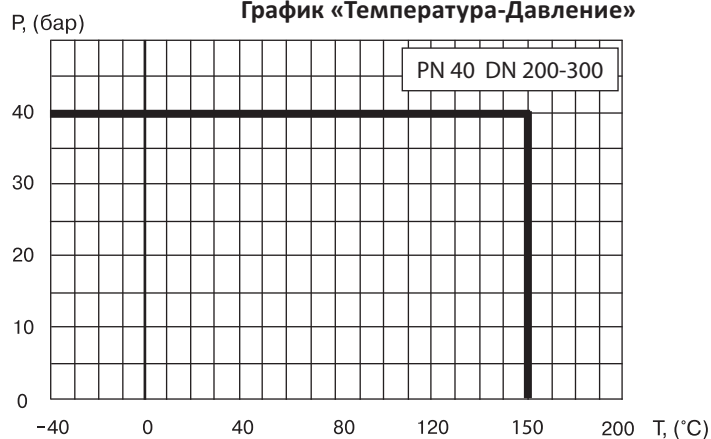
График «Температура-Давление»
