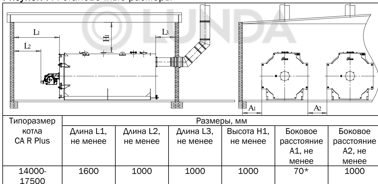
Рисунок 7. Установочные размеры
