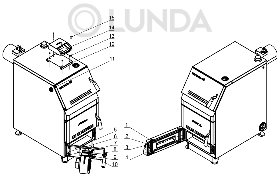
Рис.1. Установка комплекта TurboSet на котел Zota Тополь-М, Zota Тополь-ВК
