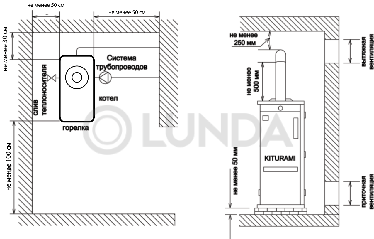
Рисунок 16. Установка котла
