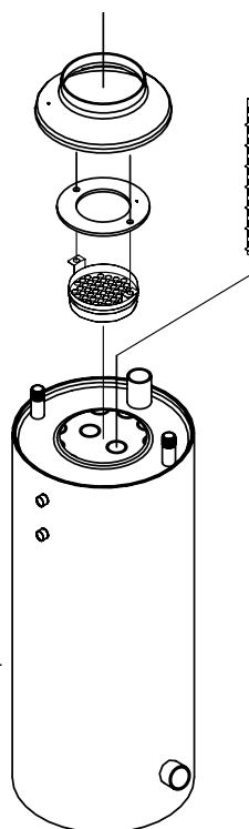
Рисунок 20. Схема доступа к жаротрубным каналам
