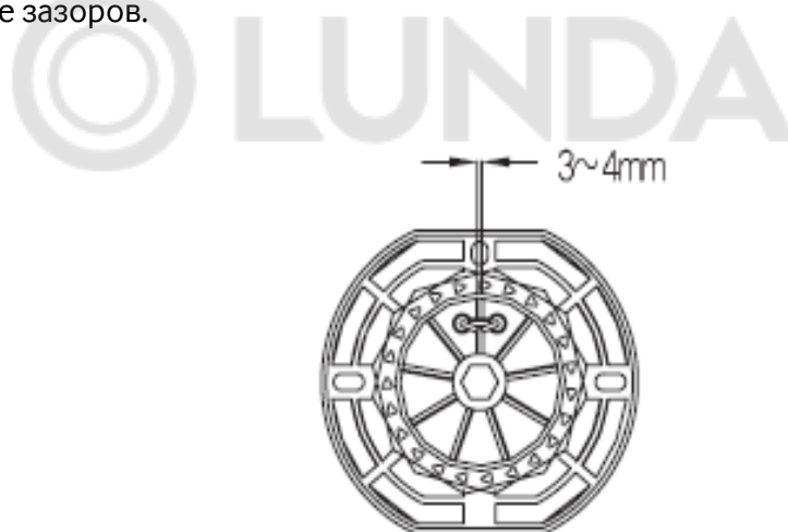
Рисунок 21. Схема регулировки системы поджига
