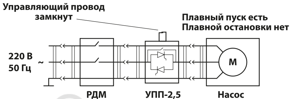
Схема 3. Подключение УПП-2,5 после механического реле давления типа РДМ
