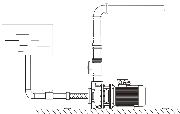
Рисунок 5 – Насос установлен ниже уровня перекачиваемой жидкости
