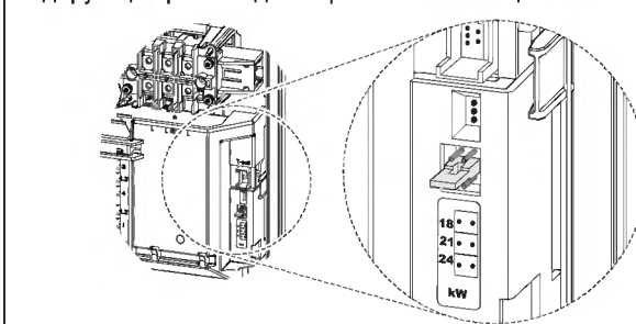
Кодирующий разъем для переключения мощности
