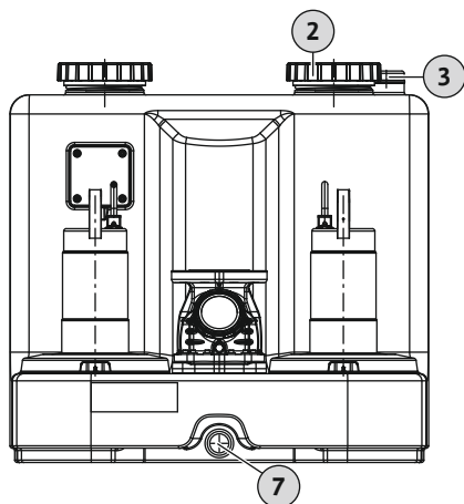
Fig. 7: Подсоединение ручного мембранного насоса
