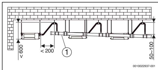
Рис. 17 Установка и габариты дренажного трубопровода с водяным насосом (мм)
