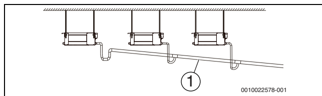
Рис. 18 Монтаж сливного трубопровода без водяного насоса
