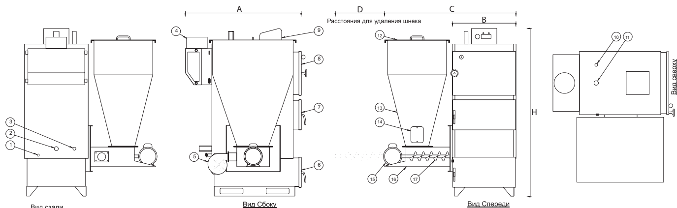
Рис. 1. Котел VLK PRK
