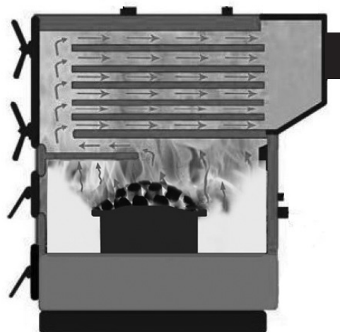
Рис. 5. Схема движения дымовых газов в трехходовом теплообменнике для котла VLK PRK 160-1500.
