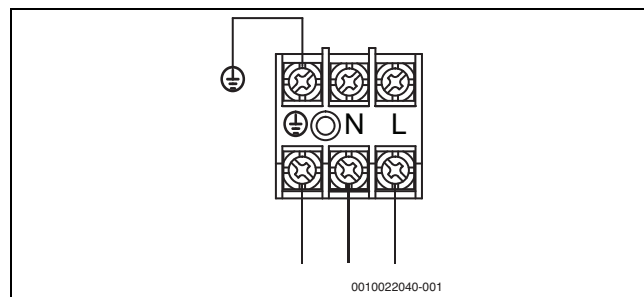
Рис. 35 Входное питание
