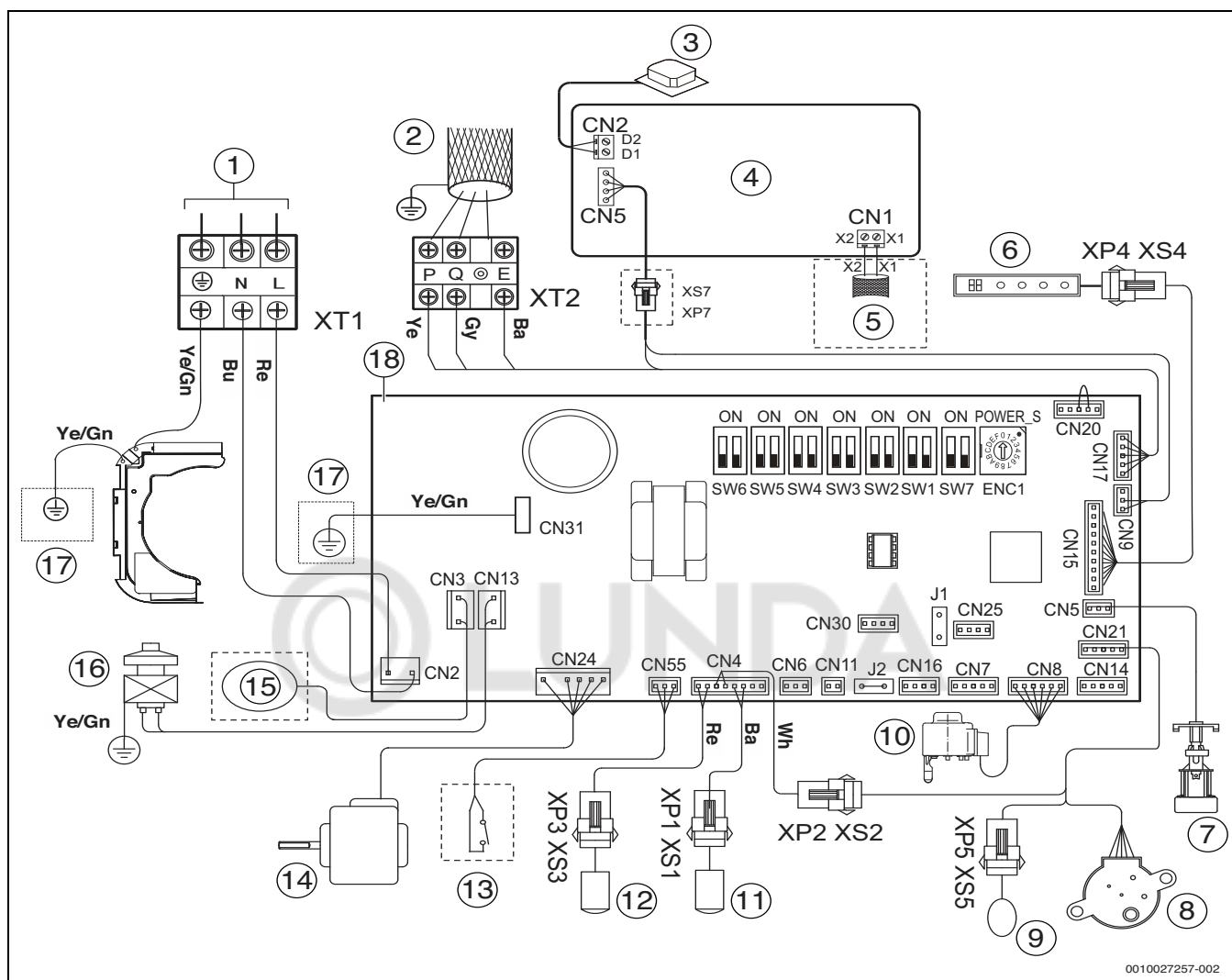
Рис. 51 Электропроводка
