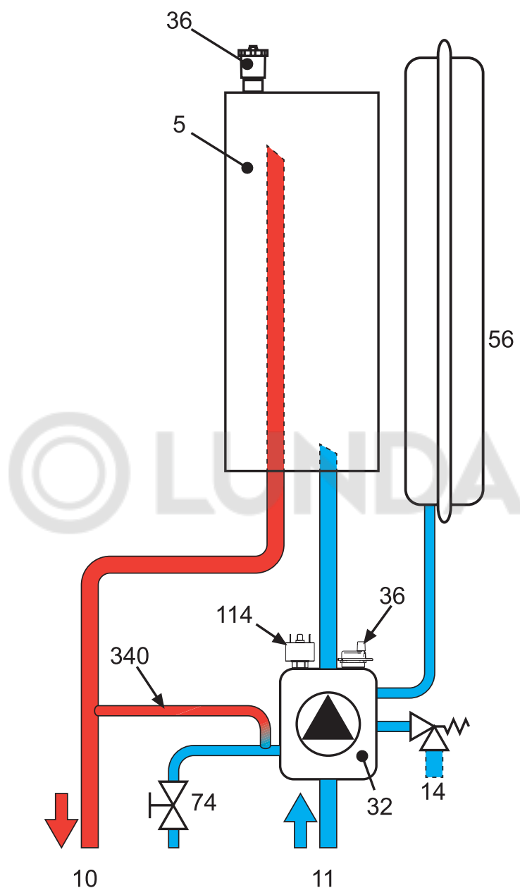
Рис. 16 Гидравлическая схема
