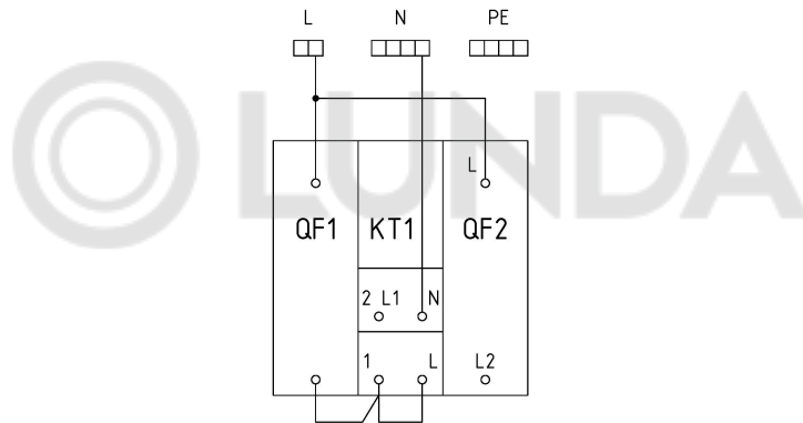
Рис. 9.2 Монтажная схема щита управления установки ЛОС 8.
