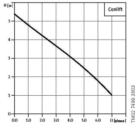
Рис. 9 График характеристики
