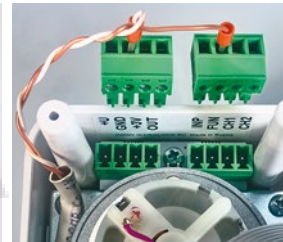
Фото 18. Подключение проводного выключателя к электроприводу
