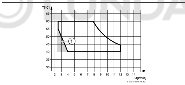
Рис. 11 Диаграмма температуры подаваемой холодной воды от +15 °С (ZWC 24)
