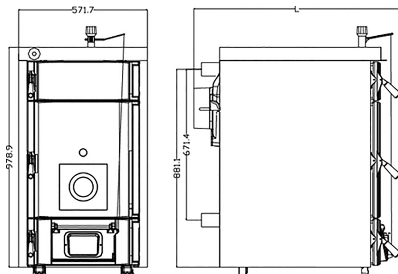
Рис. 14. Размеры котла
