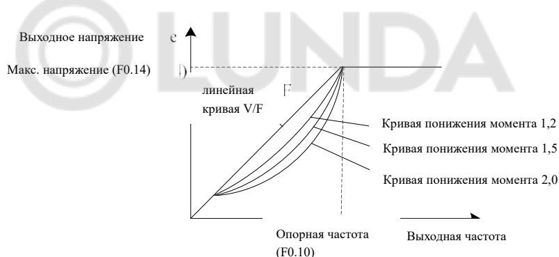
Рис. 6-8 Кривая понижения крутящего момента
