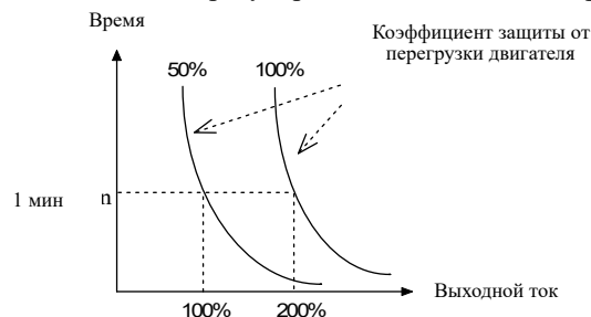
Рис. 6-27 Кривая защиты двигателя от перегрузки
