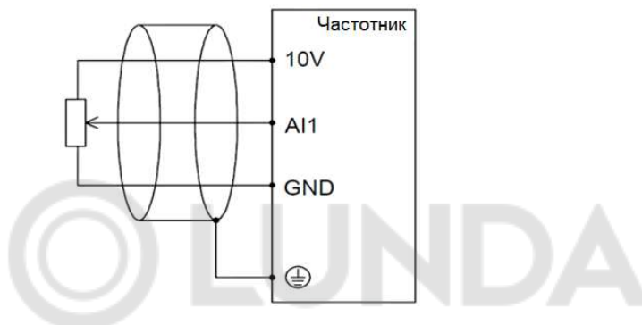
Рис. 3-14 Подключение аналоговых входов
