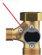
Рис. 1 б. Байпас закрыт.
