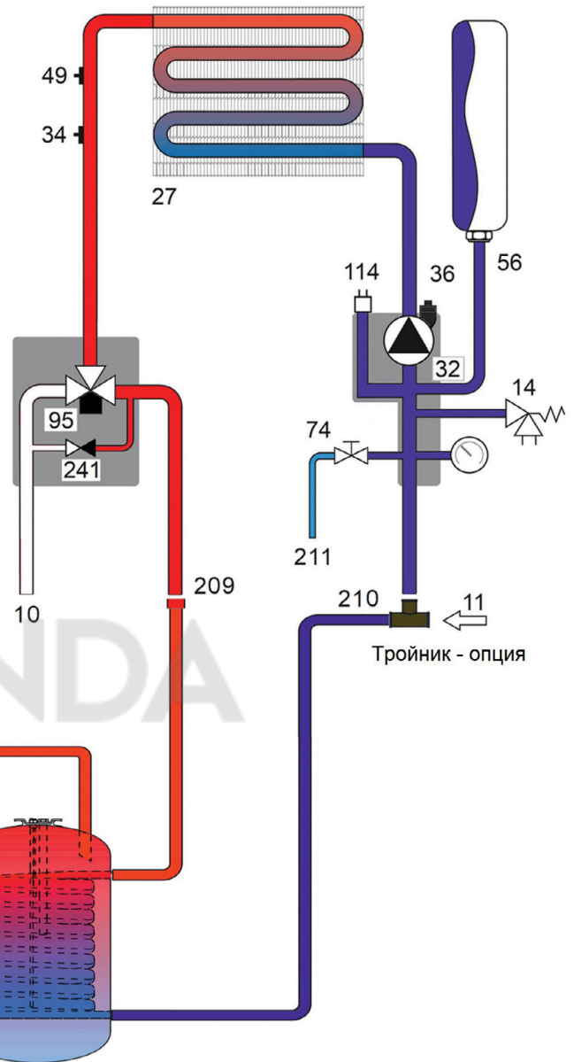
Рис. 19. Схема подключения внешнего бойлера
