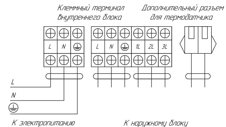
Внутренний блок
