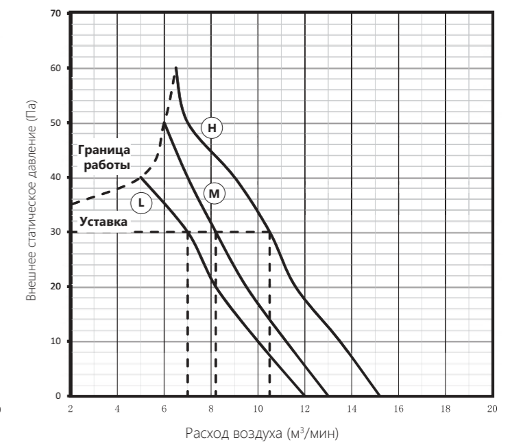
AUD-12HX4SNL (уставка 30 Па)
