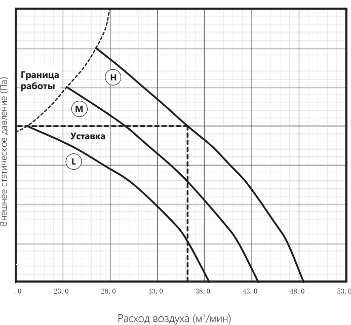
AUD-48HX4SHH (установка 80 Па)
