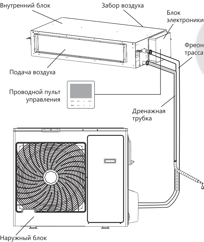
Наружный блок (типоразмер 12/18/24/36)
