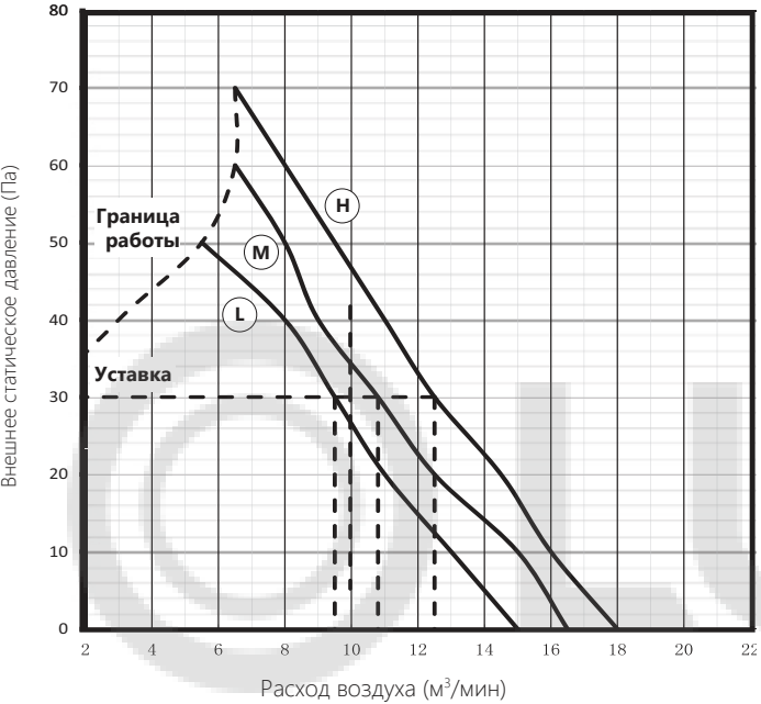
AUD-18HX4SNL1 (установка 30 Па)
