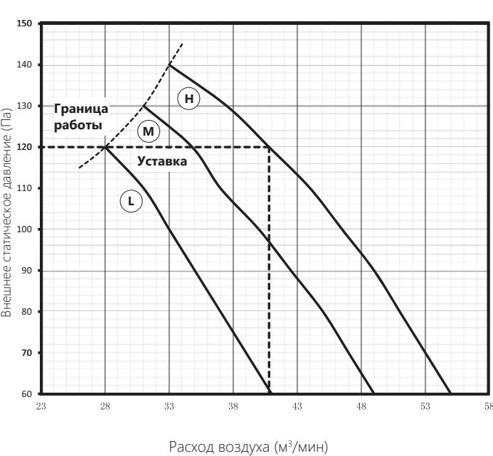
AUD-48HX4SHH (установка 120 Па)
