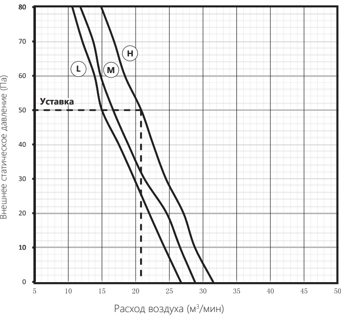
AUD-24HX4SLH1 (установка 50 Па)
