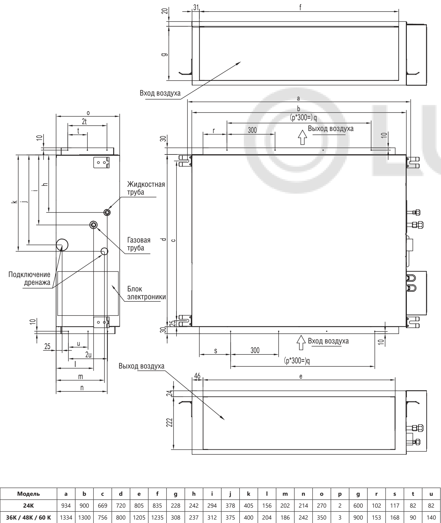
Блоки канального типа, типоразмеры 24/36/48/60
