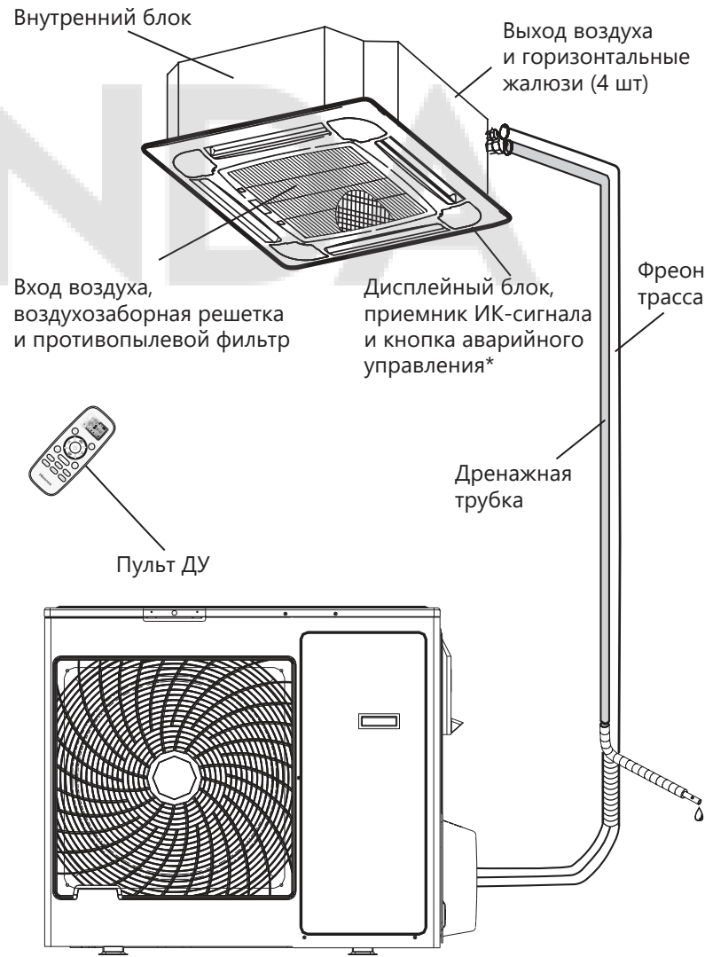
Наружный блок (типоразмер 12/18/24/36)
