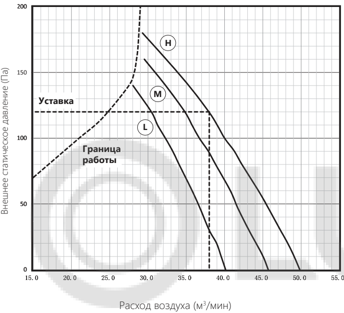
AUD-60HX4SHH (установка 120 Па)
