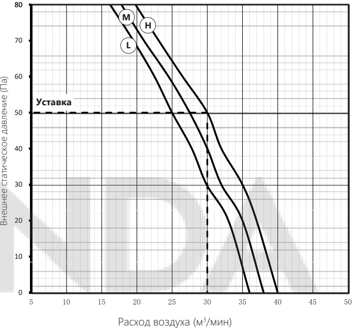
AUD-36HX4SHH1 (установка 50 Па)
