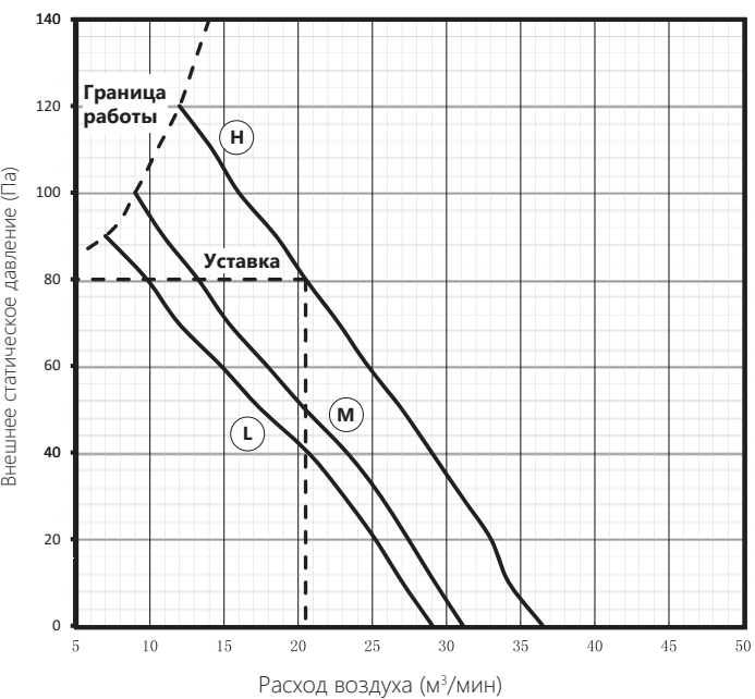
AUD-24HX4SLH1 (установка 80 Па)
