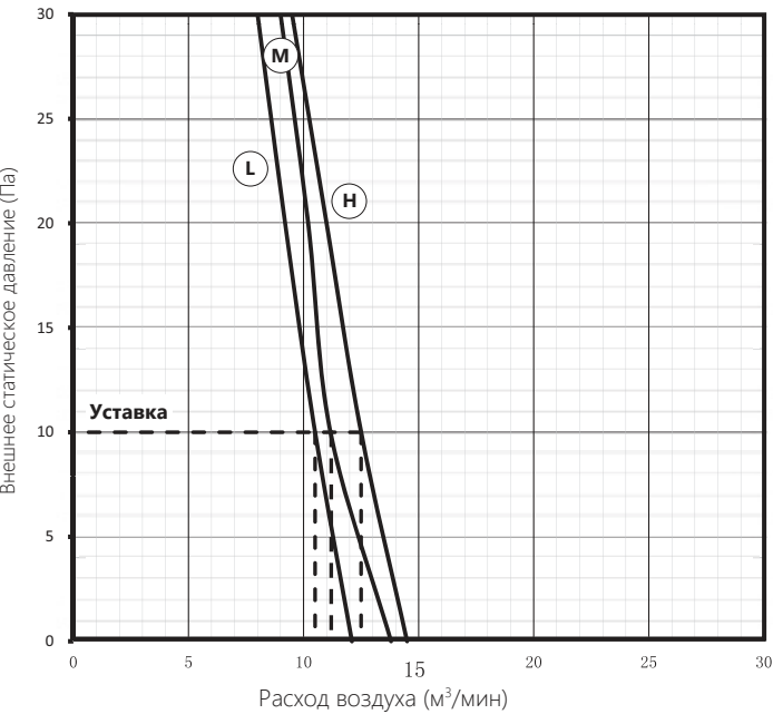
AUD-18HX4SNL1 (установка 10 Па)
