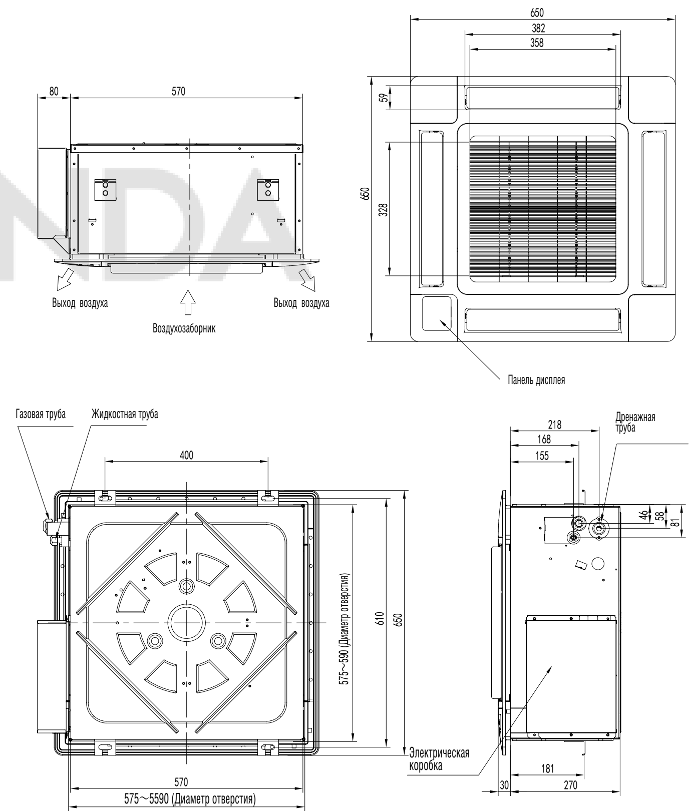
Блоки кассетного типа, типоразмеры 12/18
