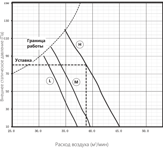
AUD-60HX4SHH (установка 80 Па)
