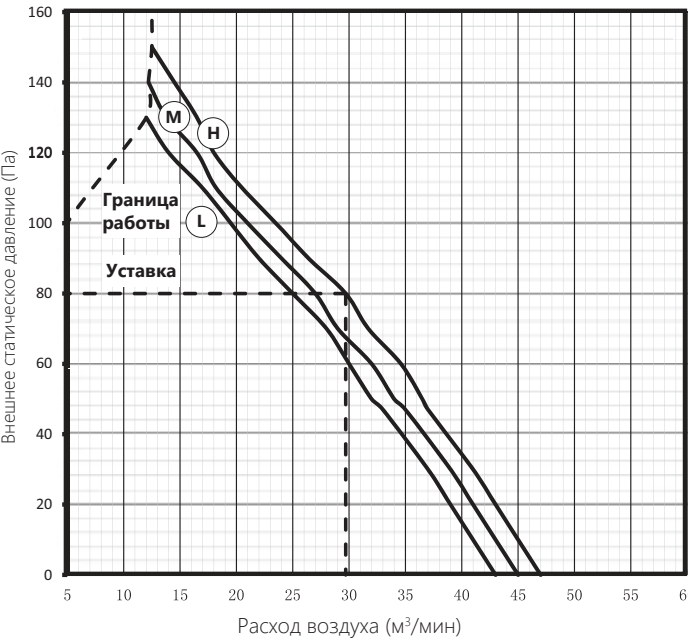
AUD-36HX4SHH1 (установка 80 Па)
