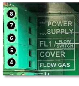
Датчик расхода: ⑤ & ⑦
