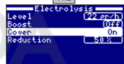
11.2 Процент сокращения выработки хлора при закрытой створке. Когда створка закрыта, нет необходимости в работе системы на 100%. Этот параметр позволяет выбрать оптимальную настройку выработки хлора.
