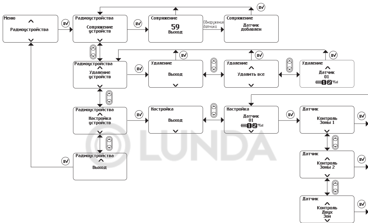
Рис. 17 Подменю “Радиоустройства”
