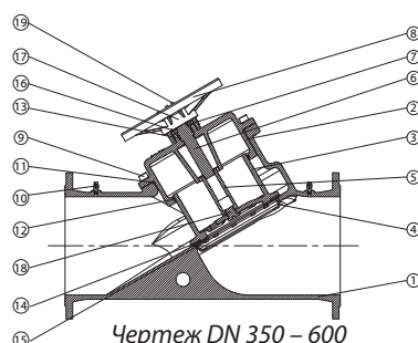
Чертеж DN 350 – 600
