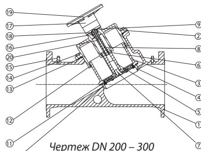
Чертеж DN 200 – 300
