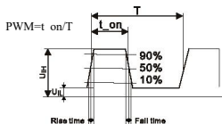
Рис. 11. Форма сигнала ШИМ
