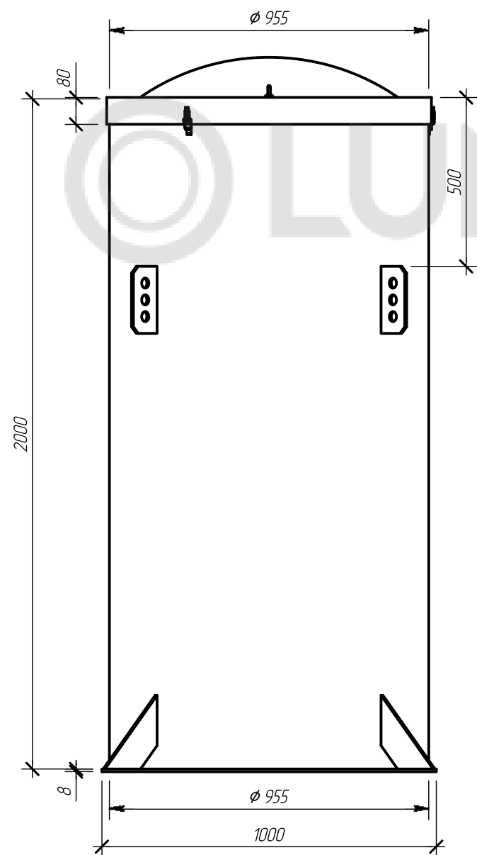
Вид спереди
