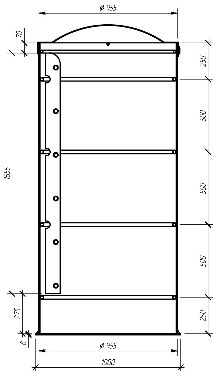
A-A (0.0625)
