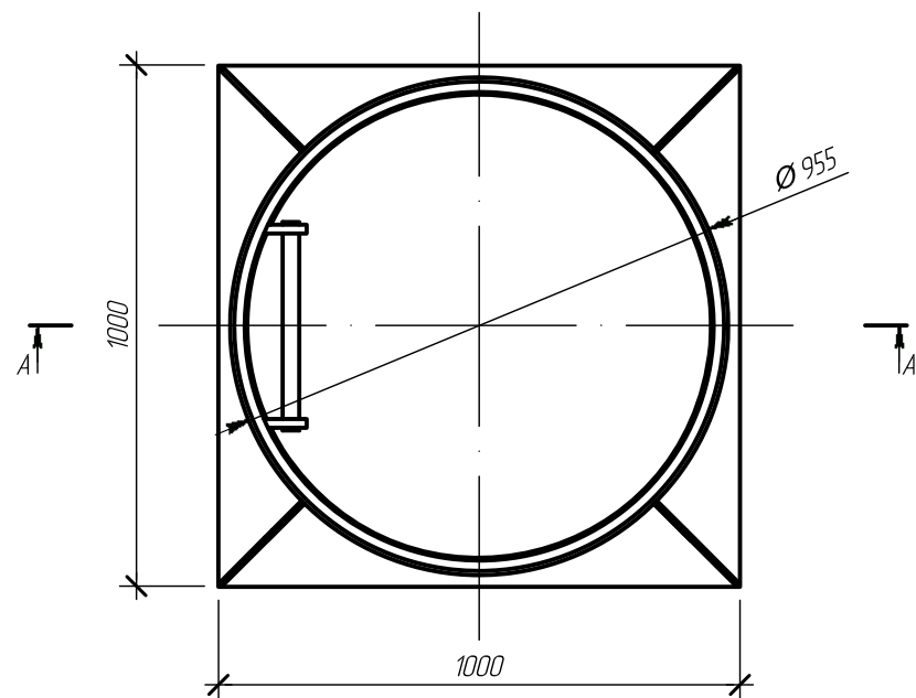
Вид сверху
