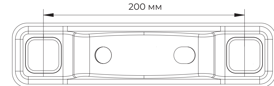
Рис. 6. Кронштейн крепления
